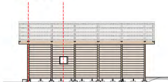
Façade OUEST Echelle: 1:100 mm
